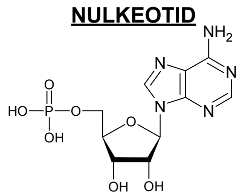
Adenosin-5-fosfát
