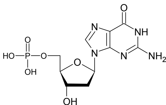
Guanosin-5-fosfát
