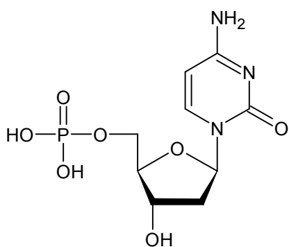
Cytidin-5-fosfát
