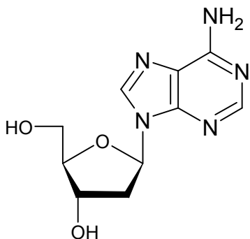
Adenosin
