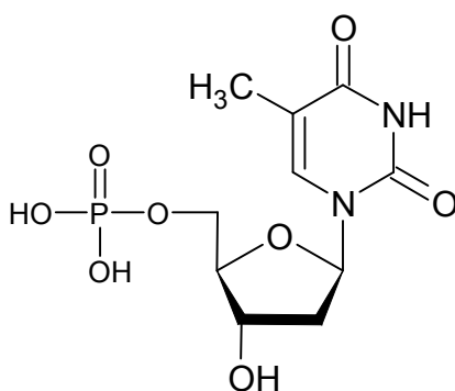
Thymidin-5-fosfát
