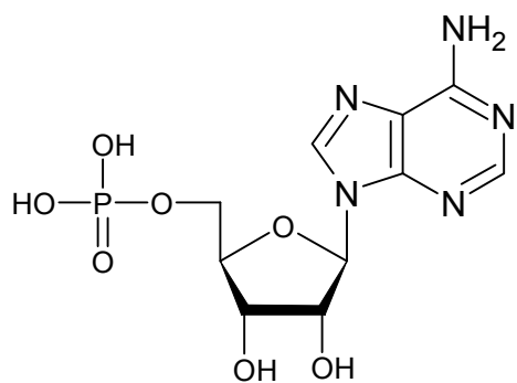
Adenosin-5-fosfát
