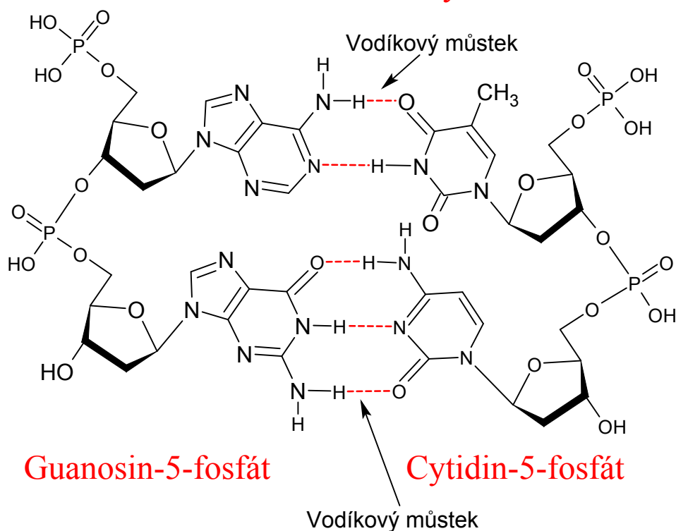
Thymidin-5-fosfát
