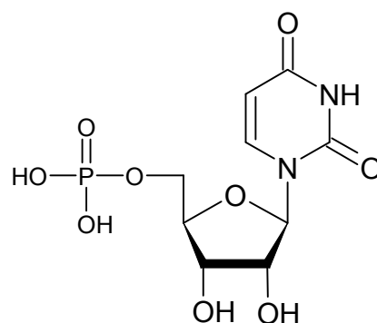
Uridin-5-fosfát
