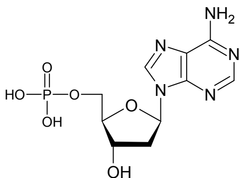
Adenosin-5-fosfát
