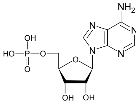
Adenosin-5-fosfát
