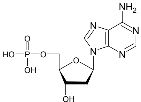
Adenosin-5-fosfát
