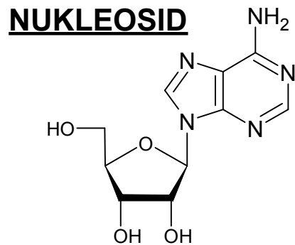
Adenosin
